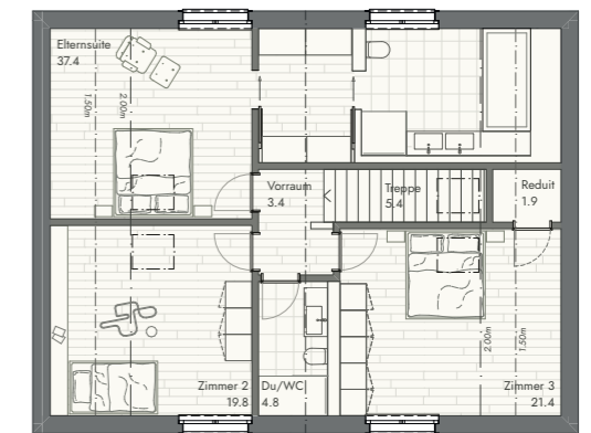
Dachgeschoss
